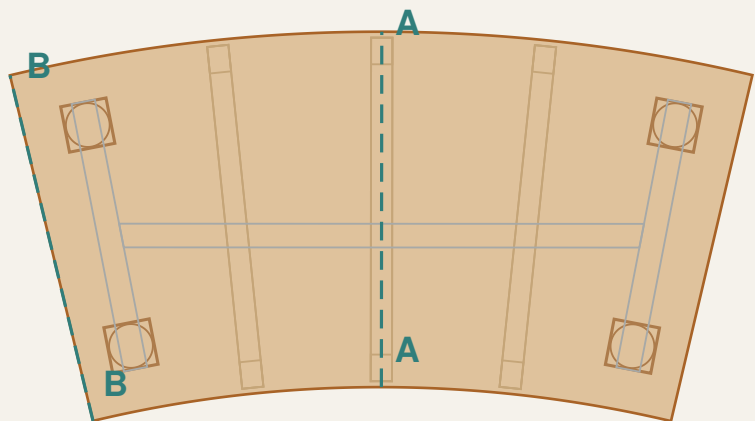
M09 / planta: dos travesaños en las estaciones de patas y un larguero central
